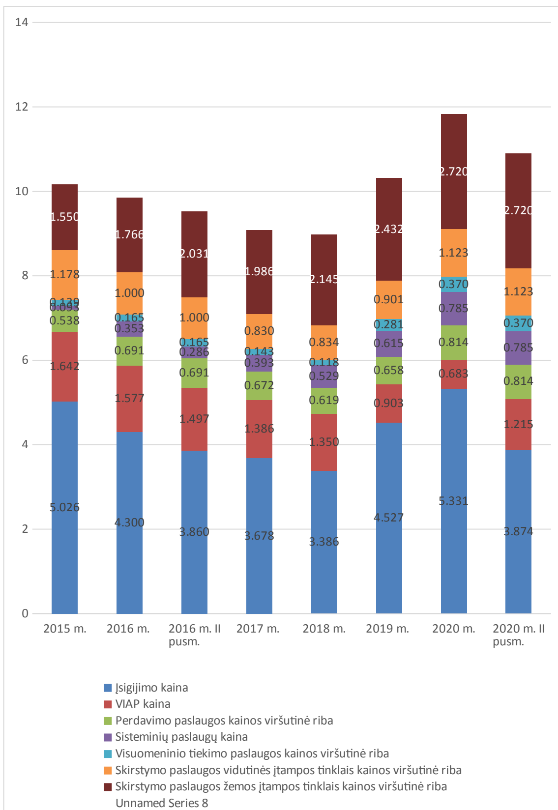
2 pav. Visuomeninės elektros energijos kainos viršutinės ribos buitiniams vartotojams, perkantiems elektros energiją iš žemos įtampos tinklų dinamika 2015–2020 metais, ct/kWh
